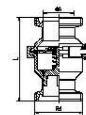
DIN check valve thread end
