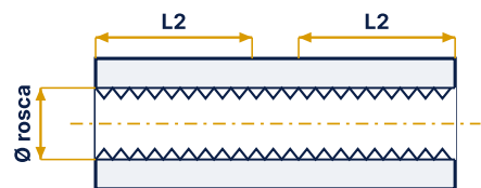
ROSCA HEMBRA NPT EN AMBOS EXTREMOS
